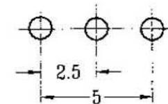
P.C.B LAYOUT
